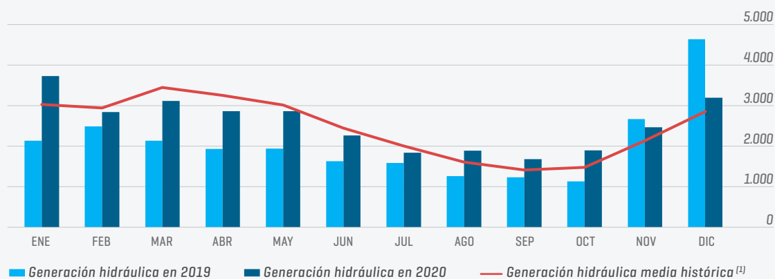
Generación hidráulica peninsular 2019-2020 comparada con la generación media GWh
